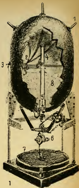
Querschnitt durch eine Mine
